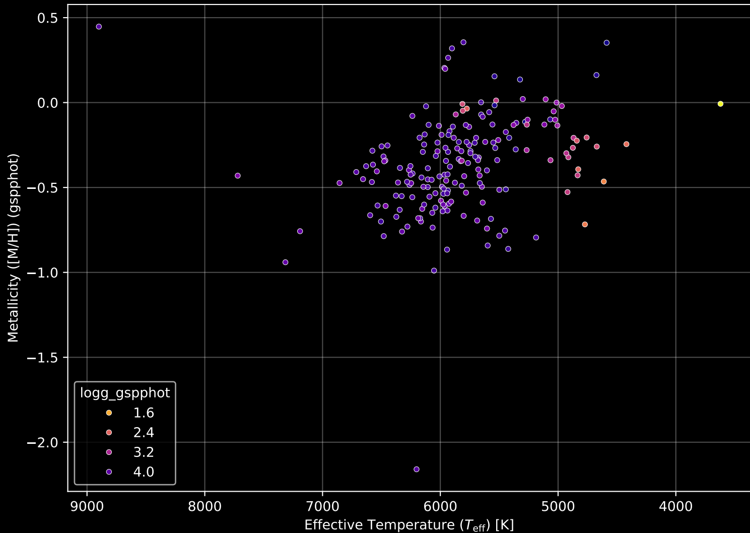
GALAH DR4 Field: [507] Stellar Population Parameters (n= 191)
