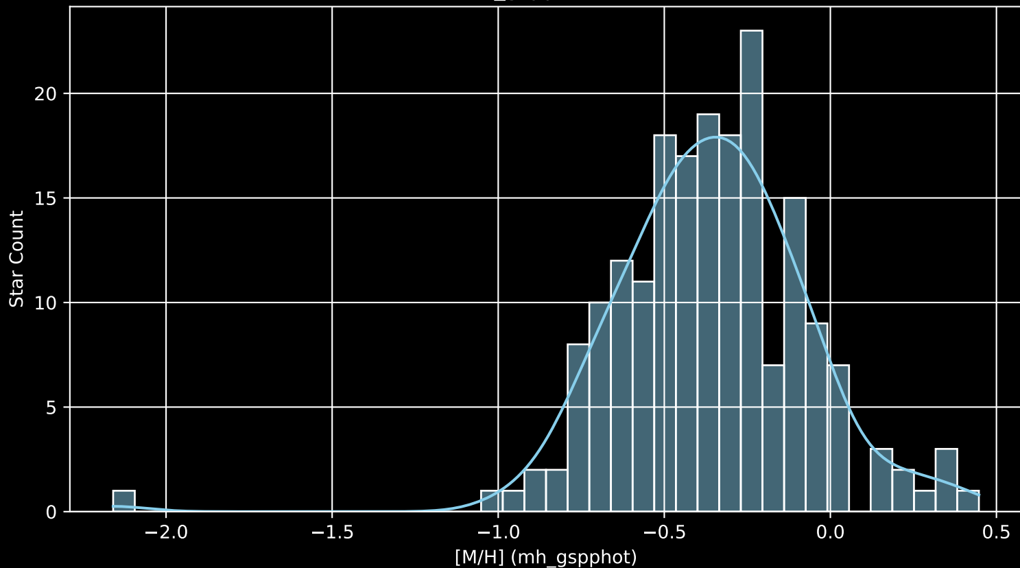
GALAH DR4 Field: [507] [M/H] (mh_gspphot) (n= 191)
