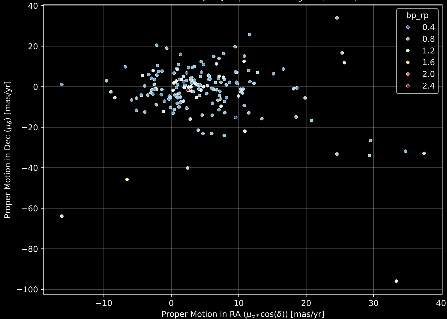
GALAH DR4 Field: [507] Proper Motion Diagram (n= 191)
