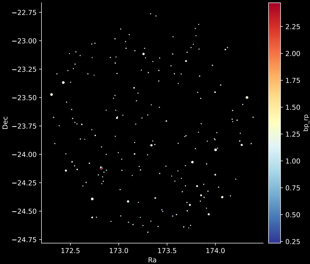
GALAH DR4 Field: [507] Stars: 191
