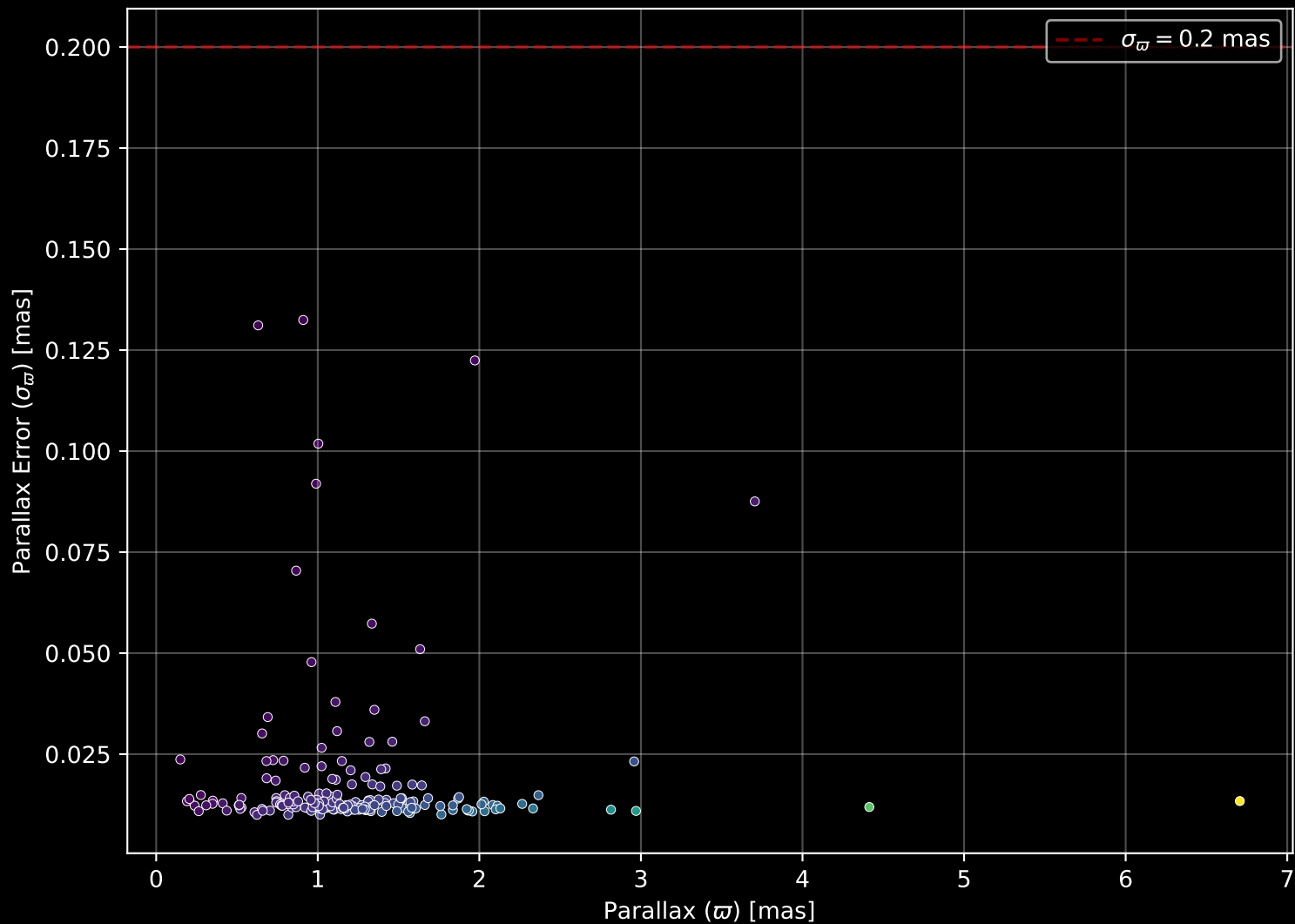
GALAH DR4 Field: [507] Parallax Quality (n= 191)
